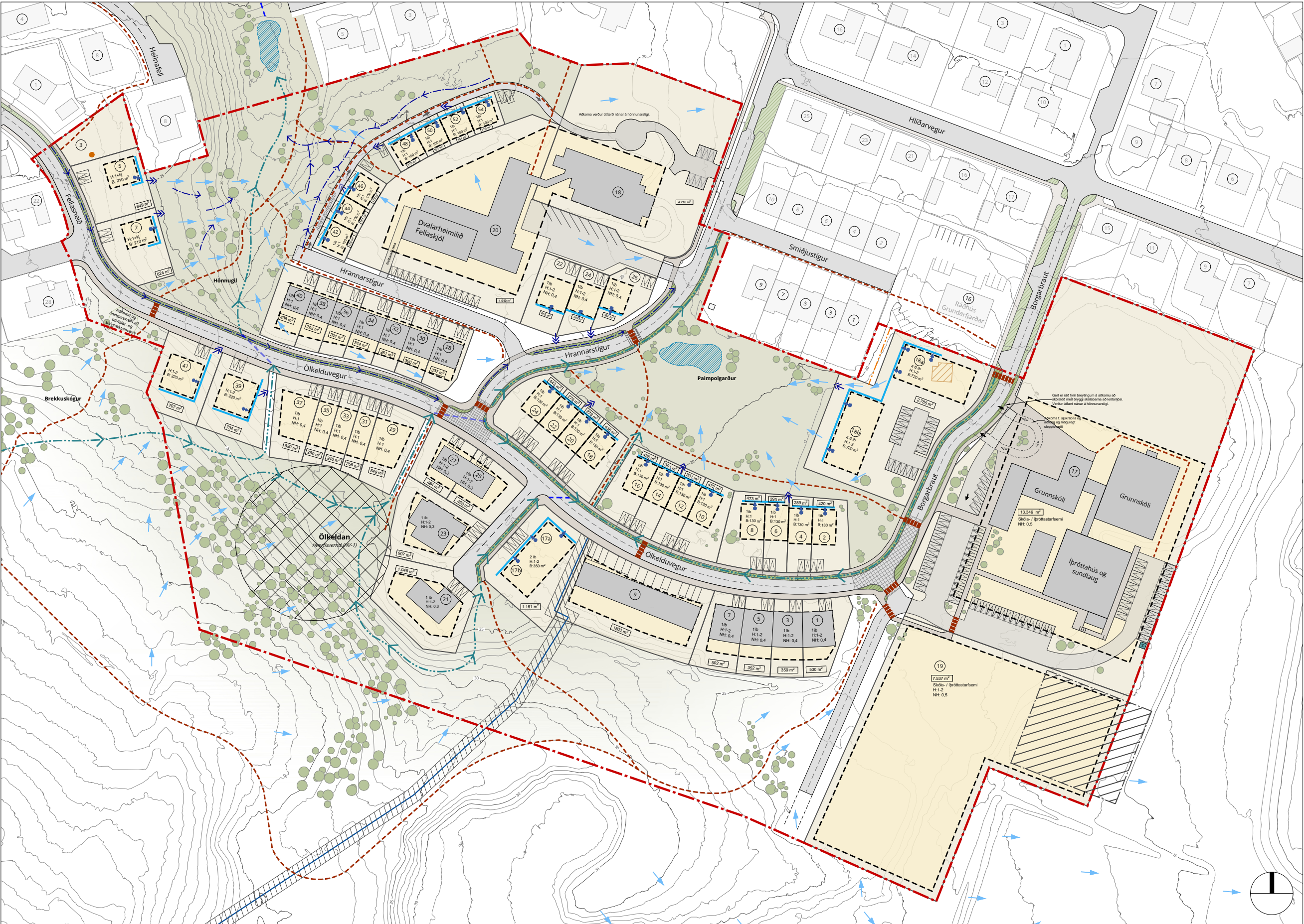
Ofanvatnsskipulag í mkv. 1:1500
