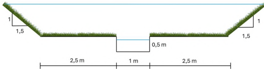
Mynd 4.12: Kennisnið fyrir árfarvegin við Gilósinn
