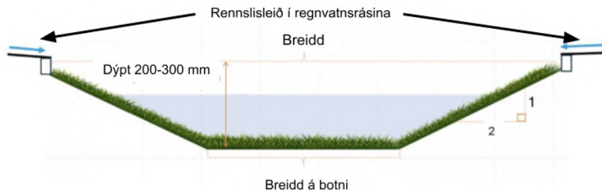
Mynd 4.8: Kennisnið fyrir dæmigerða regnvatnsrás.
